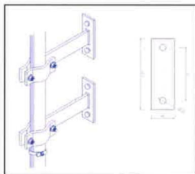
Pattes déport
